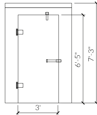
36" WIDE DOOR
