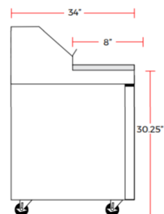
SP-SERIRS SIDE VIEW
