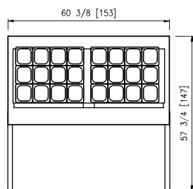
TOP NLSMP60-24
