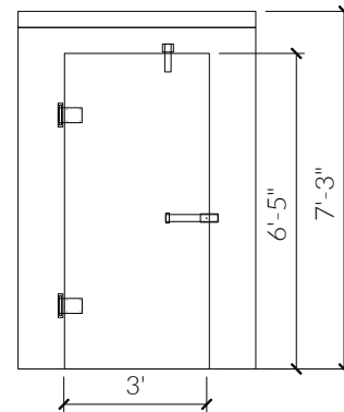
36" WIDE DOOR
